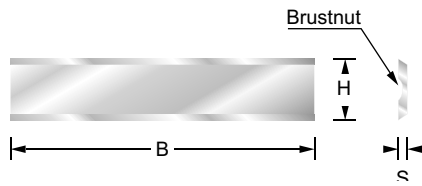
2-schneidige Wendemesser für Messerköpfe von LEITZ.
